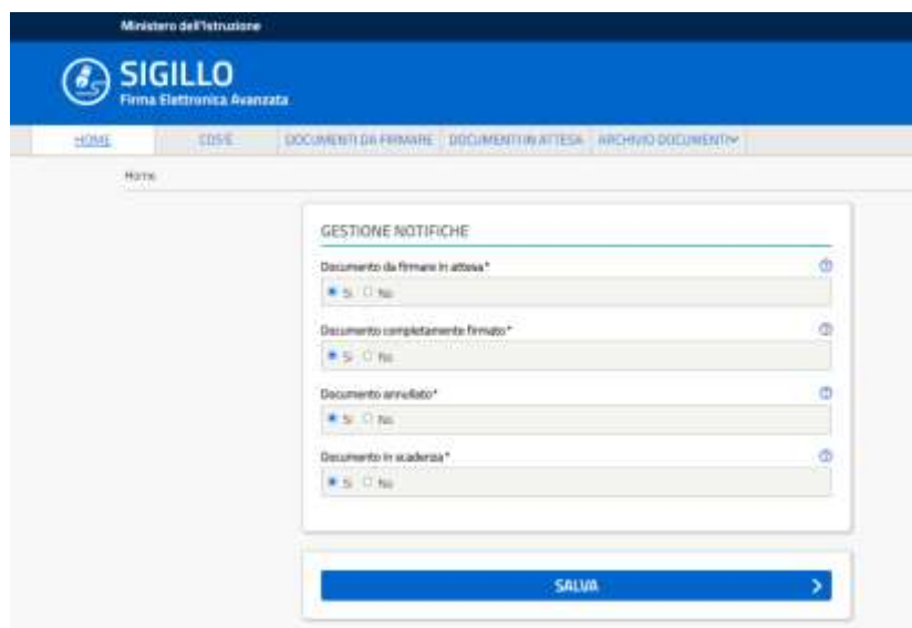
Figura 25 – Gestione notifiche
